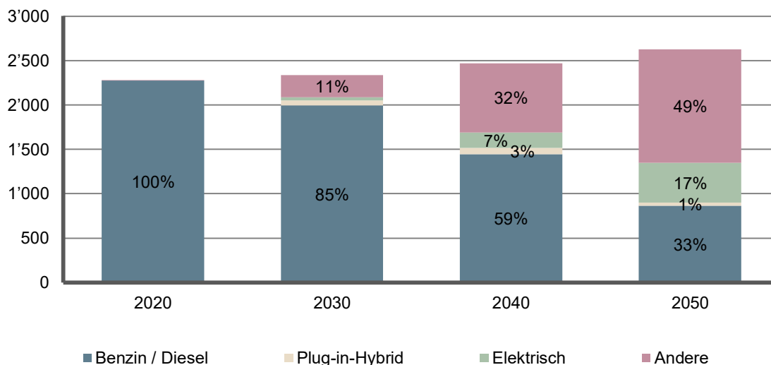
Abbildung 9 - Entwicklung schwere Nutzfahrzeuge zum Sachtransport nach Antriebsarten
